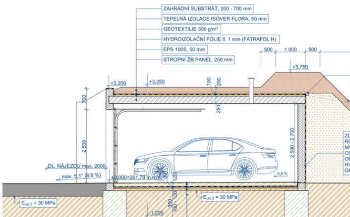
ŘEZ B-B'
